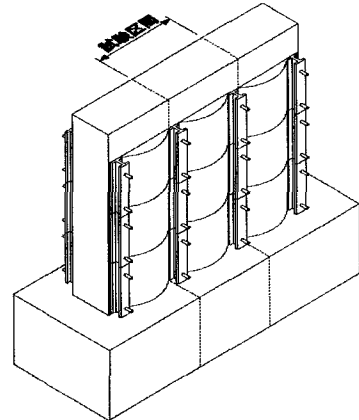
図 2.1 壁式橋脚補強概念図
