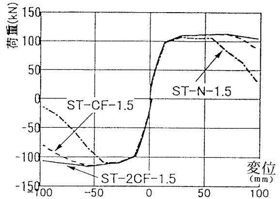
図－2 荷重－変位包絡線
