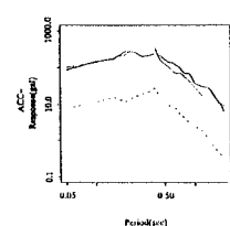
図 3 応答スペクトルの比較
