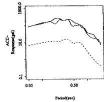
図 5 図 4 の波形の応答スペクトルの比較
