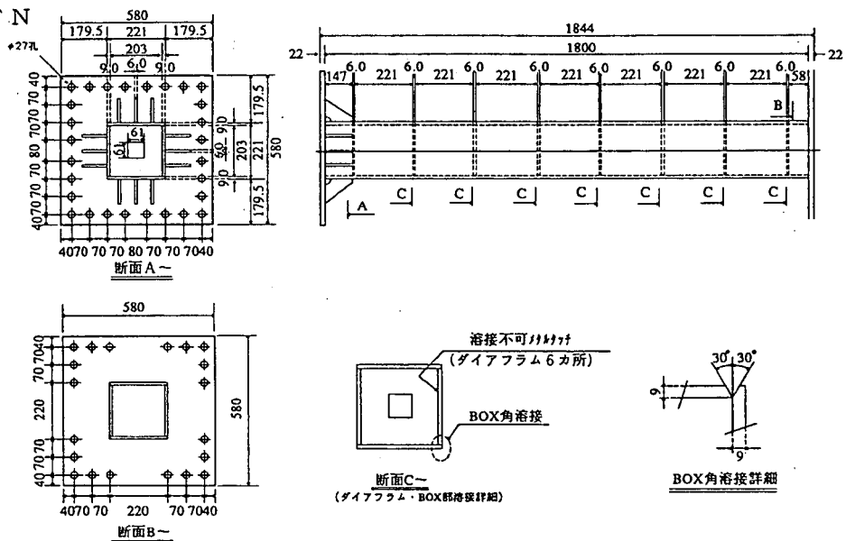
図9-4 橋脚モデルの形状と溶接ディテール
