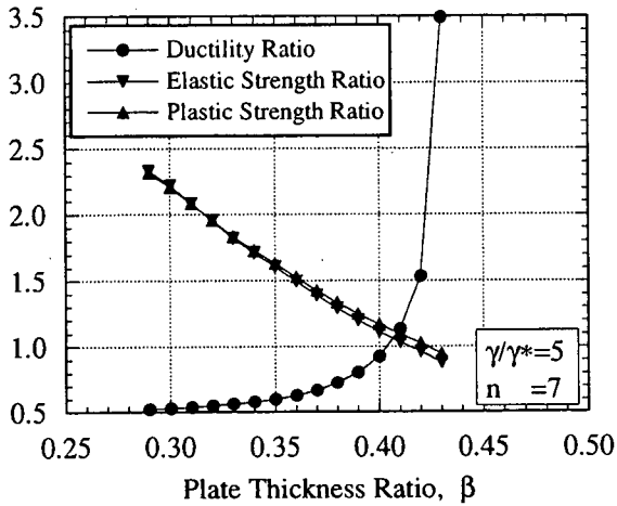
図9-15 板厚比との関係
