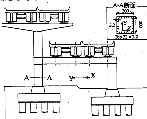
図9-1 試設計で対象とした橋脚一般図
