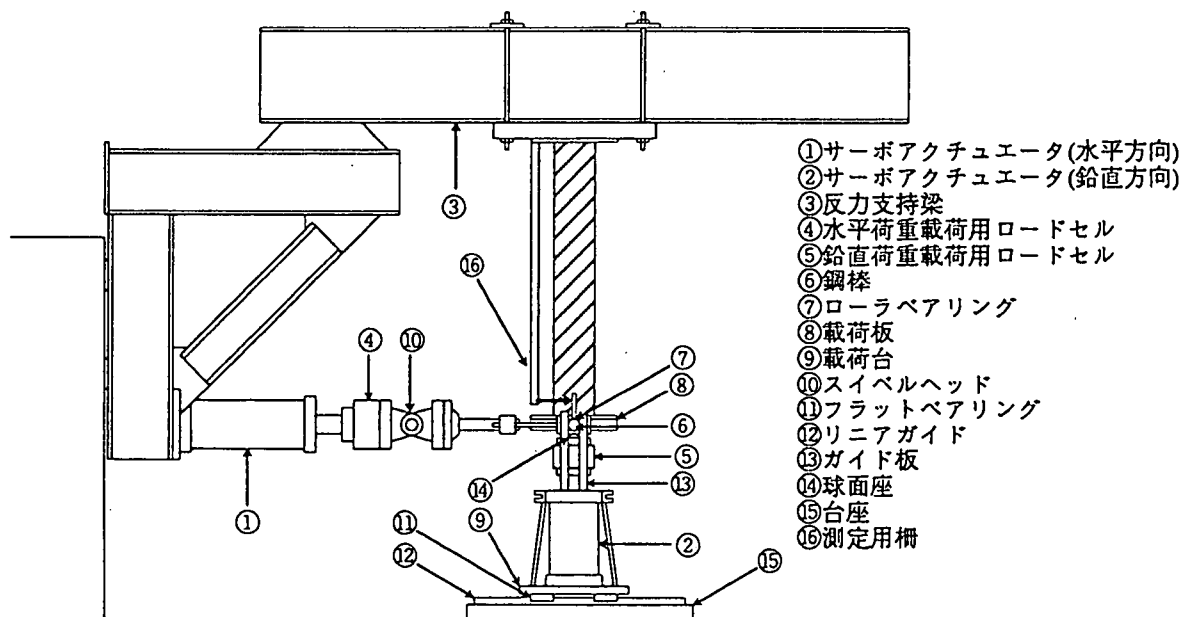
図9-5 載荷装置全体図
