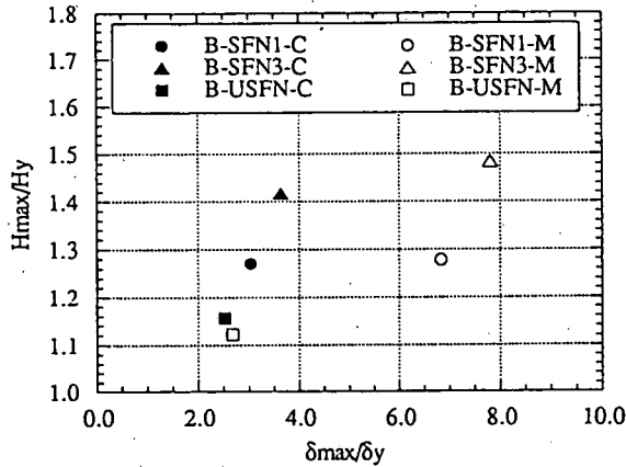
図9-10 強度と変形能の比較
