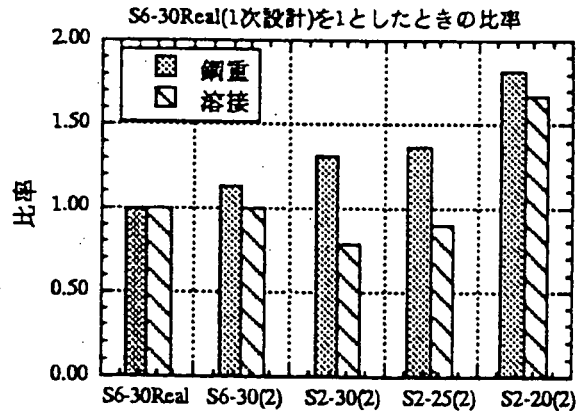
図9-3 基準断面に関する比率
