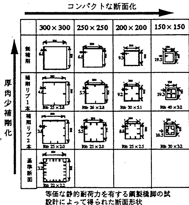
図9-2 主な検討断面ケース
