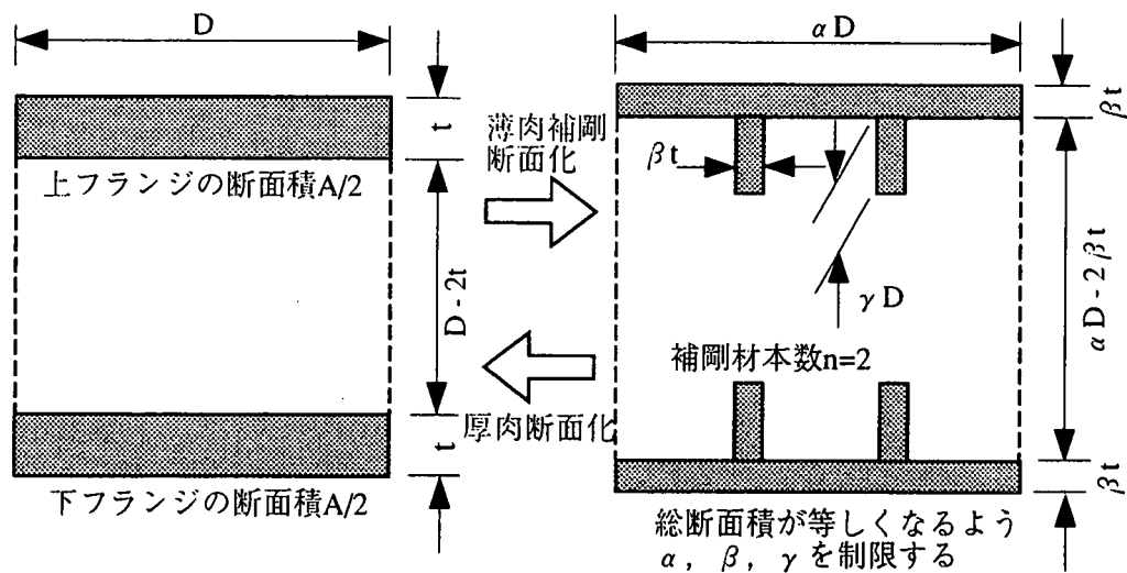
図9-14 ダブルフランジモデル
