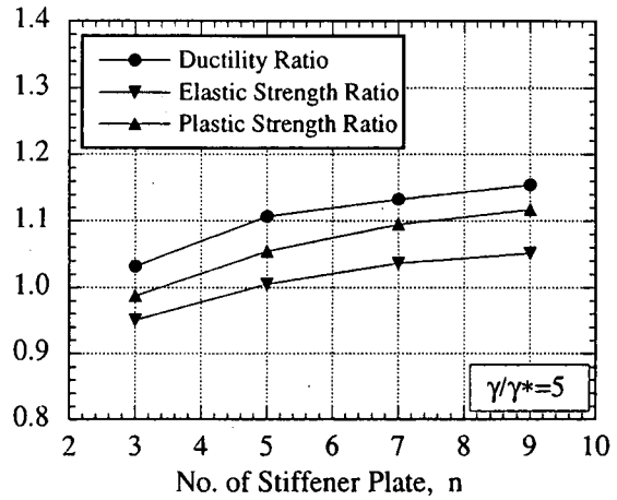
図9-16 補剛材本数との関係
