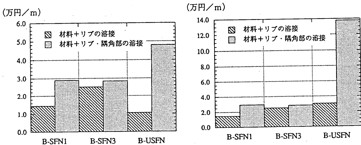
図9-13 単位長さあたりのコスト比較結果
