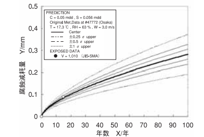
腐食予測曲線図
