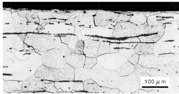
1925年 完成のリベット接合橋梁の造塊法による鋼の結晶組織
