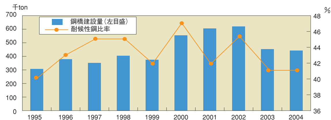
米国における鋼橋建設量と耐候性鋼が鋼橋全体に占める割合 [日本の耐候性鋼比率22%~33%(2004~2006)]
