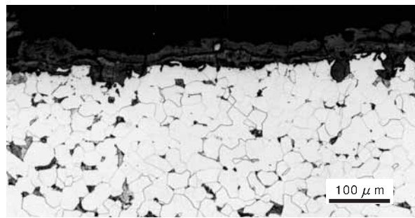
現代の溶接構造用鋼材の結晶組織
