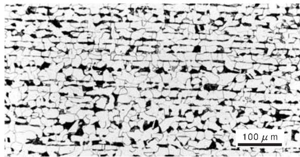
最近のTMCP鋼の結晶組織
