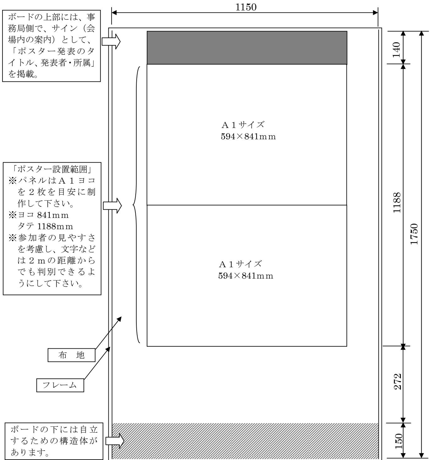
図—1 ボード寸法図とポスター仕様可能範囲
