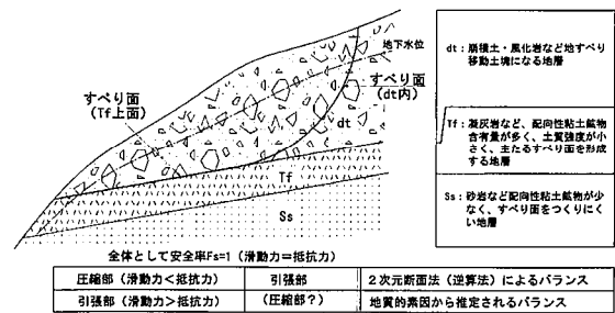
図一 3 2次元断面法(逆算法)による1円弧1直線型地すべり滑動力・抵抗力バランス
