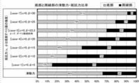
周縁部を考慮した地すべり安全率による土質調査情報から求められた滑動力・抵抗力の割合と周縁部の比率
