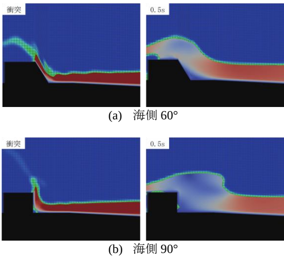
図-5 流速分布
