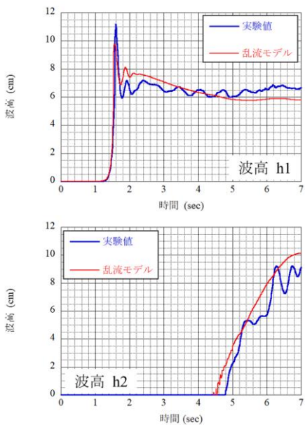
図-3 波高の比較
