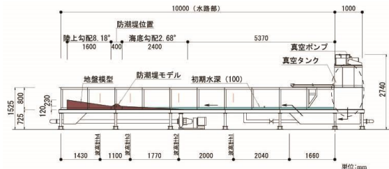
(a) 実験で使用された水路
