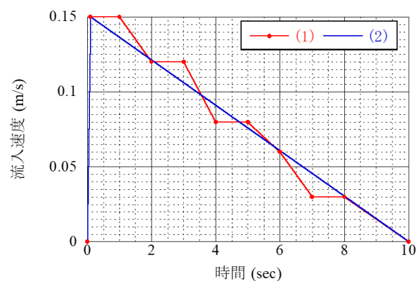
図-2 流入速度 (時刻歴)
