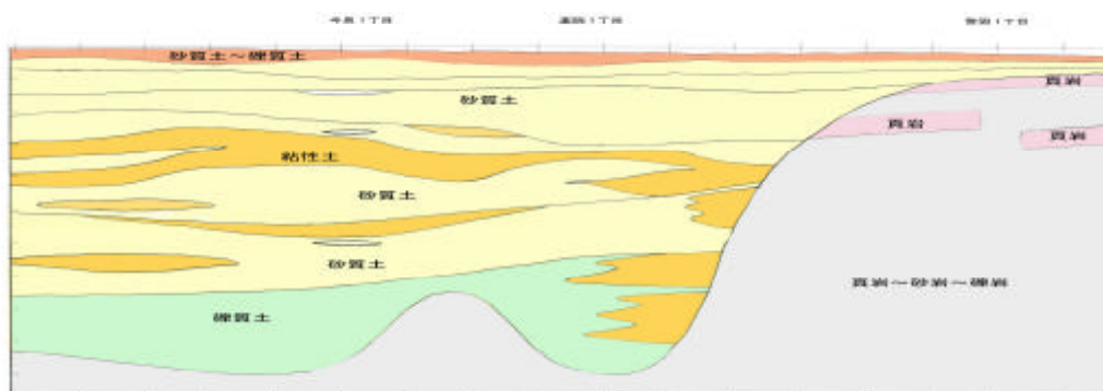
図-2.8 想定地質断面図
