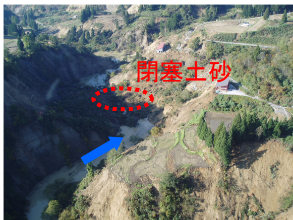
写真-7 南平地区河道埋塞状況（芋川流域）
