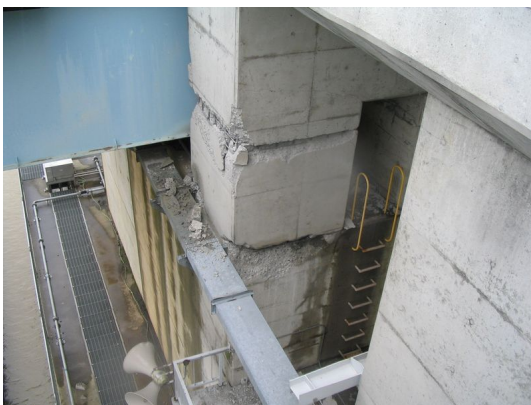
写真-5 信濃川 30.0km 妙見堰 (損傷した部位の詳細。コンクリートが剥落し、鉄筋が露出している。)
