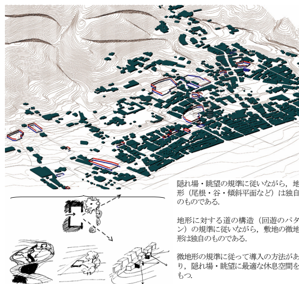
図-14 対象地域全体における系と特徴の階層
