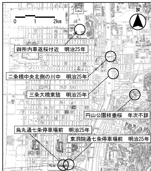
図-1 初期の電灯設置箇所（資料をもとに筆者作成）
