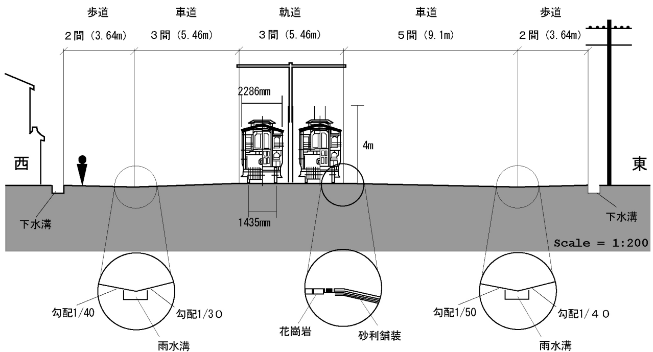
図-11 拡築後丸通断面図（『明治後期産業発達史資料第464巻』をもとに筆者作成）
