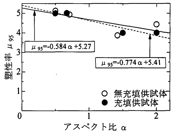
図3 塑性率とアスペクト比の関係
