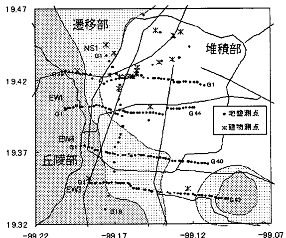
図-1 メキシコシティ市街地の測点位置
