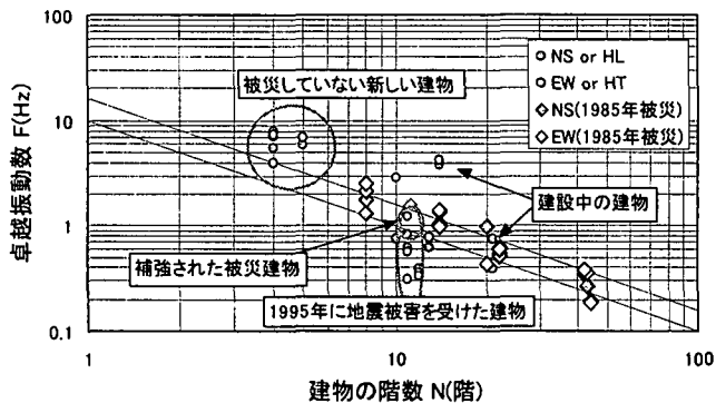
図-7 測定した建物の卓越振動数 F_b と階数 N の関係
