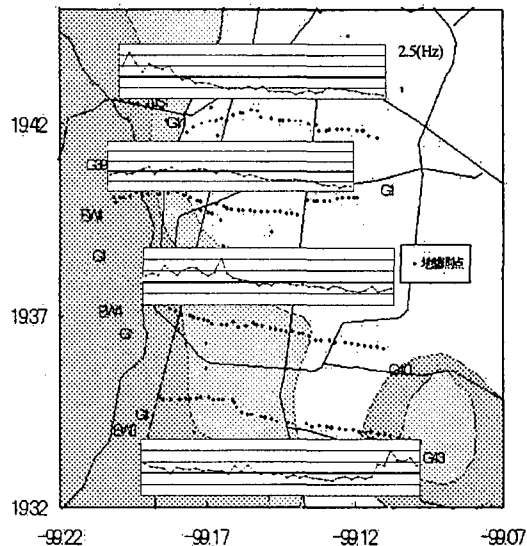
図-4 地盤区分上の卓越振動数 F_g の分布
