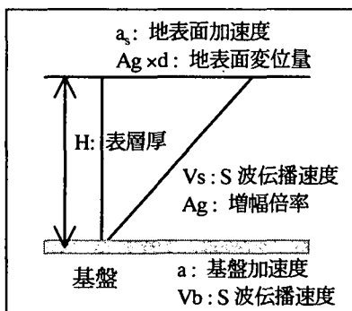
図-2 表層地盤と基盤の振動に関する模式図
