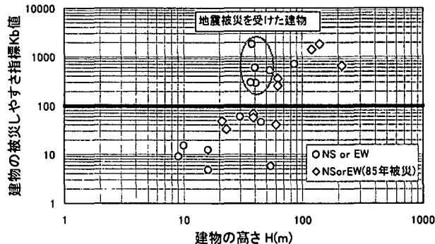
図-8 建物の被災しやすさ指標 K_b 値と建物の高さの関係
