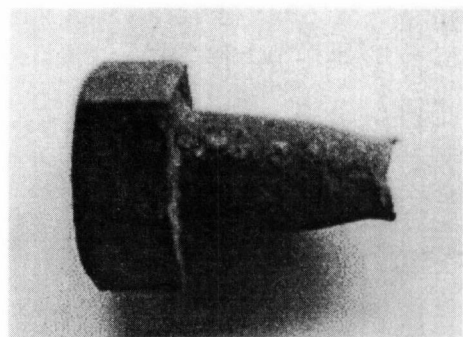
写真-1 破断した受付ボルト
