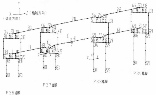
図-4 H橋全体系解析モデル
