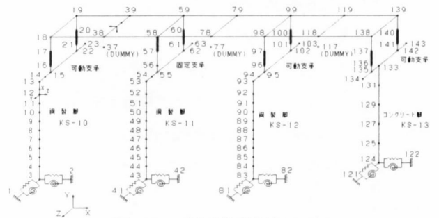
図-3 K橋全体系解析モデル
