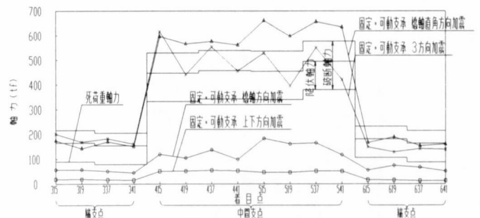
図-5 H橋解析結果
