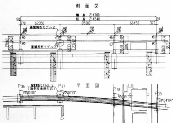
図-2 H橋一般図
