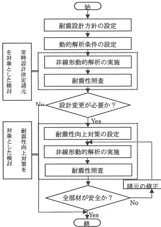
図-1 橋梁の耐震設計フロー
