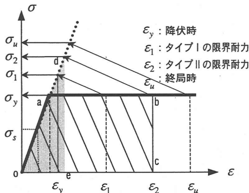
図-2 エネルギー一定則による弾性応答への換算
