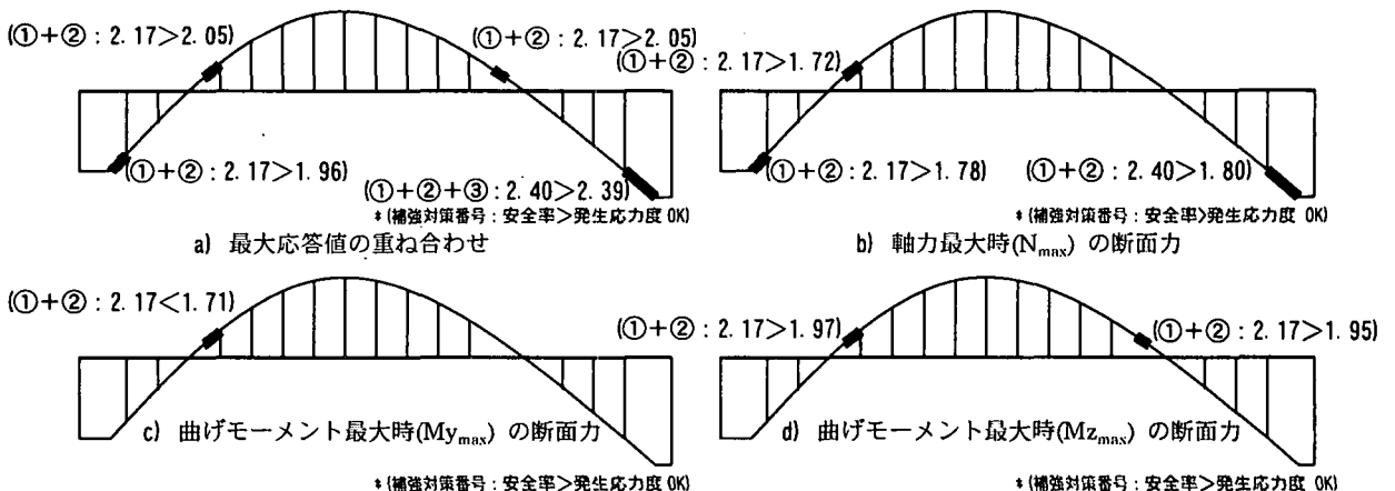
図-7 耐力が不足するアーチ部材と対策 (橋軸直角方向、タイプII加振時)
