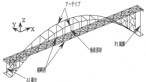
図-3 橋梁の3次元骨組モデル
