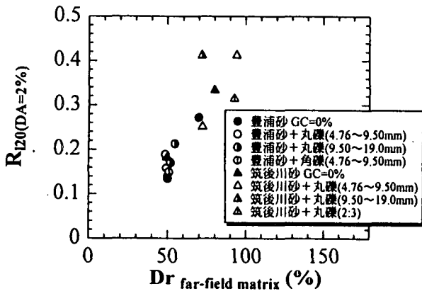
図-7 液状化強度比と Dr_{\text{far-field matrix}} の関係
