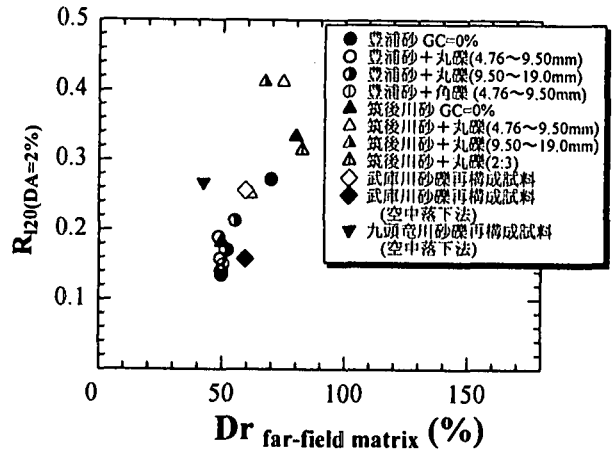
図-8 液状化強度比と Dr_{\text{far-field matrix}} の関係
