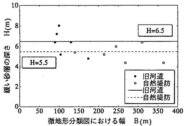
図-6 微地形の幅と実際の堆積砂層の深さの関係
