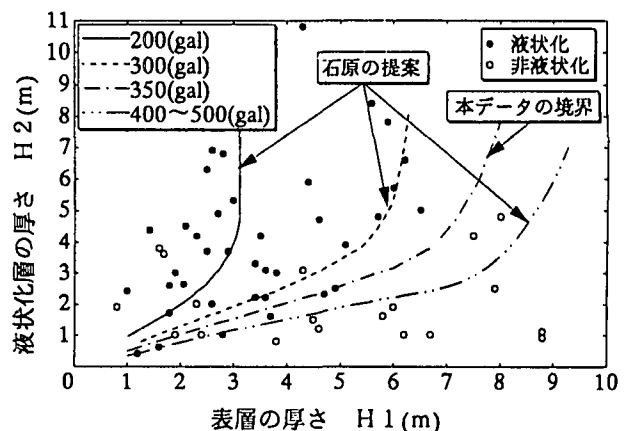
図-3 液状化・非液状化層厚と地表での液状化発生の関係
