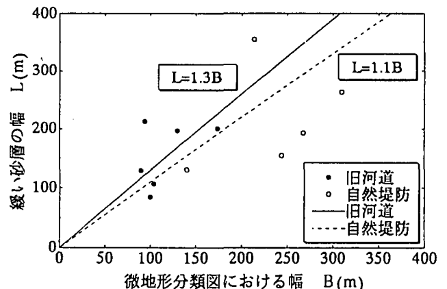
図-5 微地形の幅と実際の堆積砂層の幅の関係
