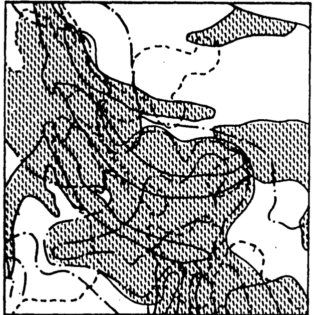
図-12 レベル2地震動での液状化予測
