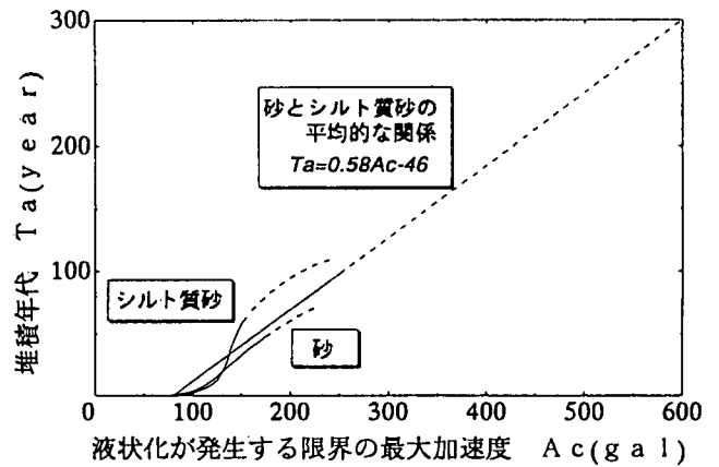
図-7 液状化が発生する最大加速度と堆積年代との関係
