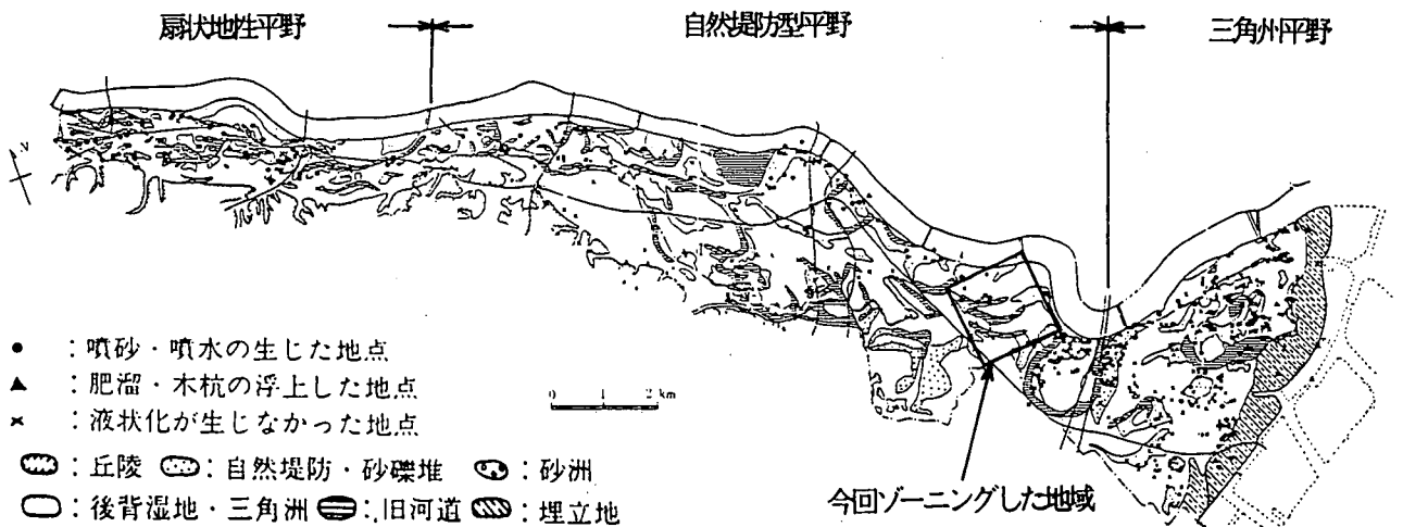
図-1 川崎市の液状化地点および微地形分類 1)
