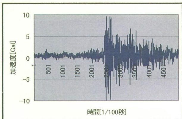
図7 1998.1.14 地震データ(港区港南)
