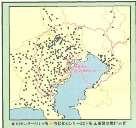
図10 現状のSIGNAL・SIセンサー配置図
