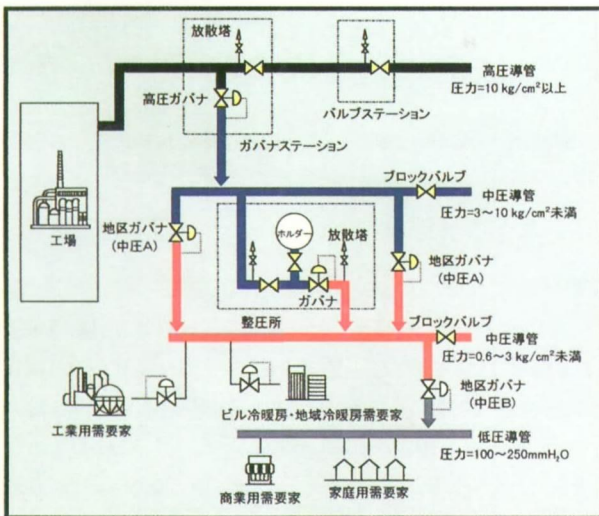
図2 東京ガス供給システムの概要
