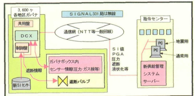
図13 新リアルタイム防災システム(SUPREME)の構成
