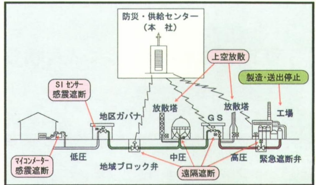
図3 大地震時の緊急遮断システム
