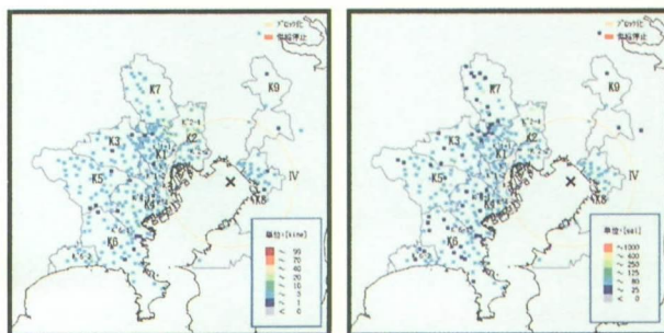
図14 1998.8.29 東京湾地震におけるSI値・加速度分布
