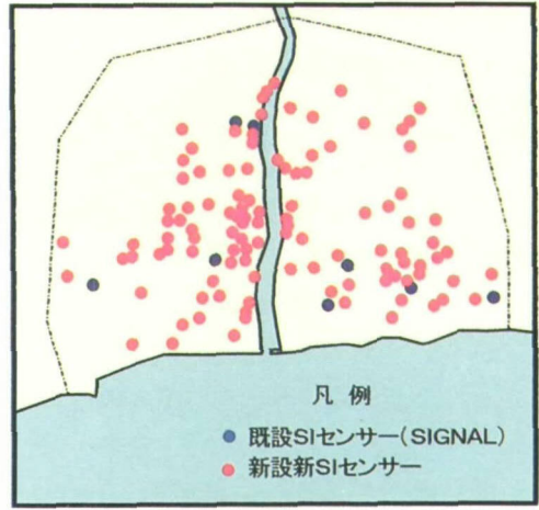
図11 湘南地区における新SIセンサー配置図
