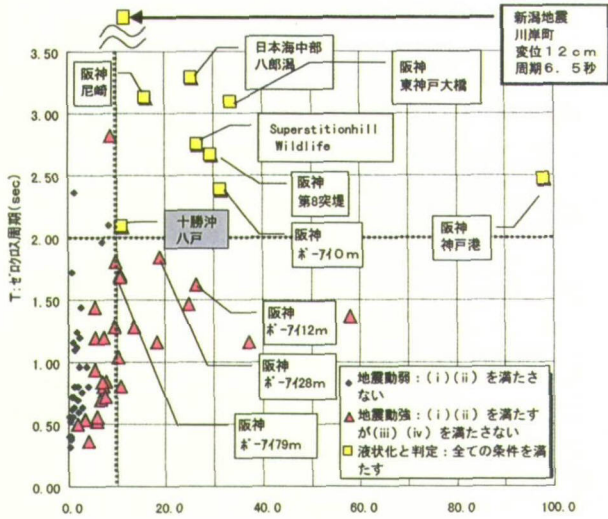
図9 液状化判定結果
