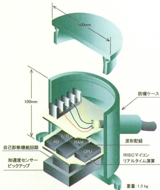
図6 新SIセンサー
