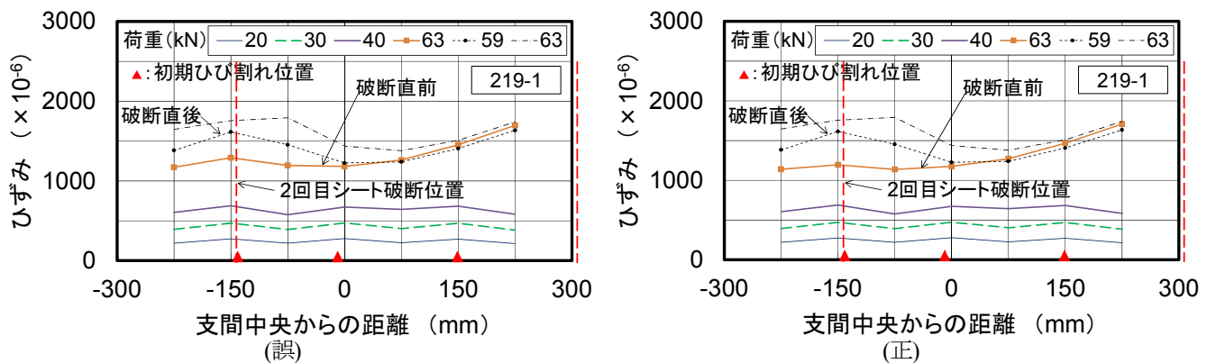
p. 1006 図-6 静的載荷試験における主鉄筋の軸方向ひずみ分布 (b) 供試体 219-1
