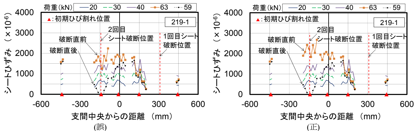
p. 1004 図-4 静的載荷試験におけるひずみゲージによるシートの軸方向ひずみ分布 (b) 供試体 219-1
