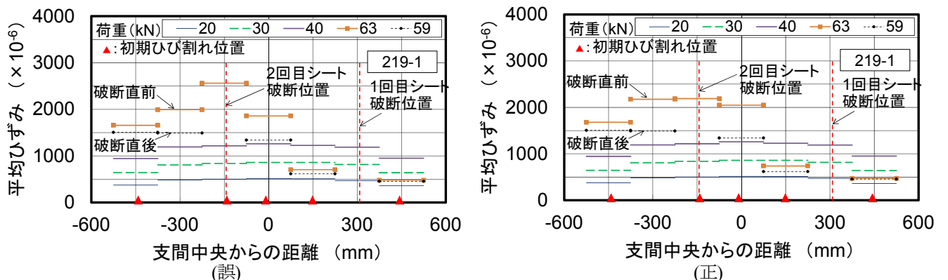
p. 1005 図-5 静的載荷試験におけるパイ型変位計による下縁の軸方向平均ひずみ分布 (b) 供試体 219-1
