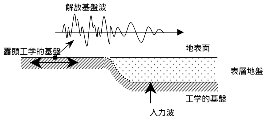
図 2.6-1 地盤応答解析の概要
