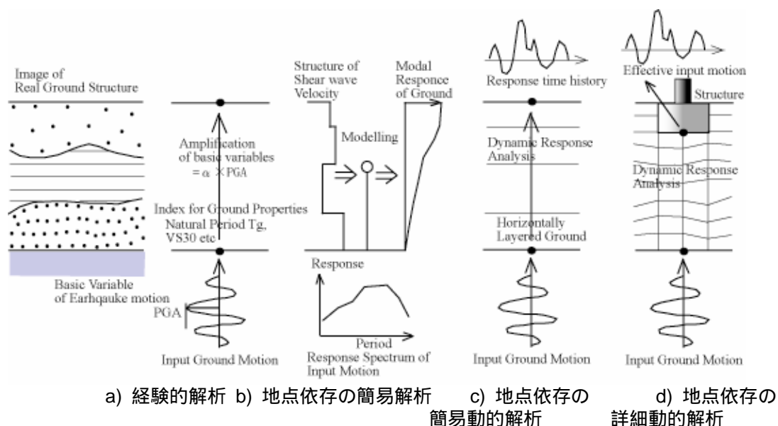
図 2.6-2 地盤応答解析法の概要
