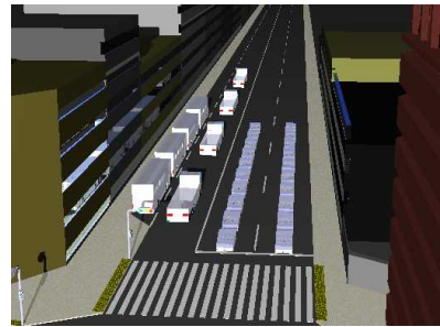
図8:改善後の第1車線使用イメージ図
