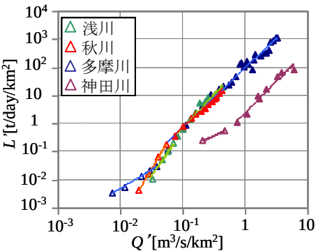
図2 比土砂輸送量 L' と比流量 Q' の相関図 （白抜き：低流量時，黒塗り：高流量時）
