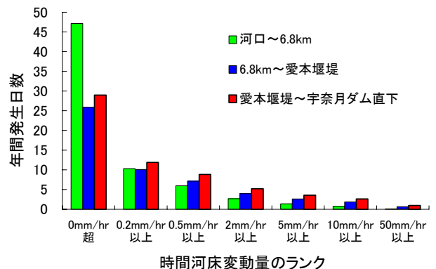
図-7 時間河床変動量の絶対値のランクと発生頻度
