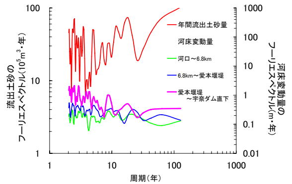
図-5 宇奈月ダムからの年間流出土砂量とダム下流区間の年間河床変動量絶対値の経年変化のスペクトル
