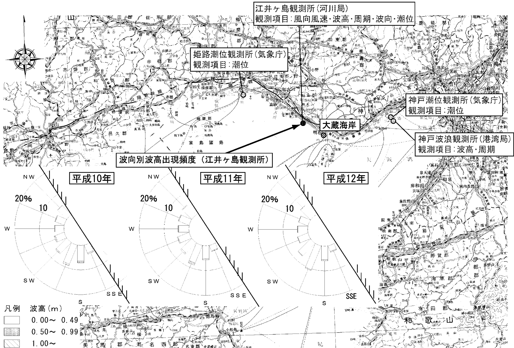
大蔵海岸周辺の観測所位置と江井ヶ島観測所における波向の出現頻度
